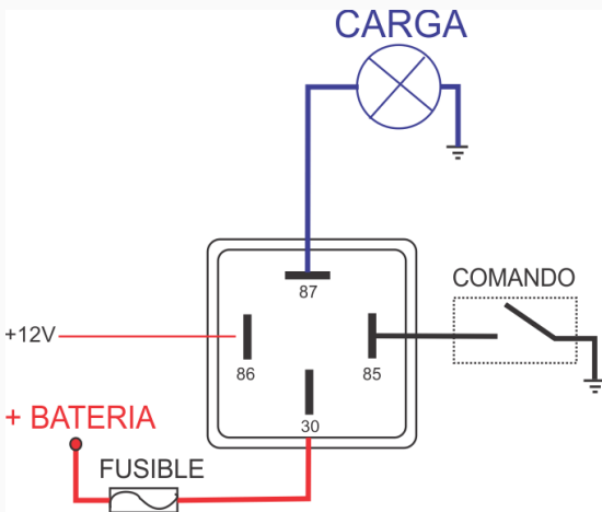
DIAGRAMA ORIENTATIVO
