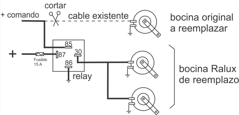
DIAGRAMA ORIENTATIVO
